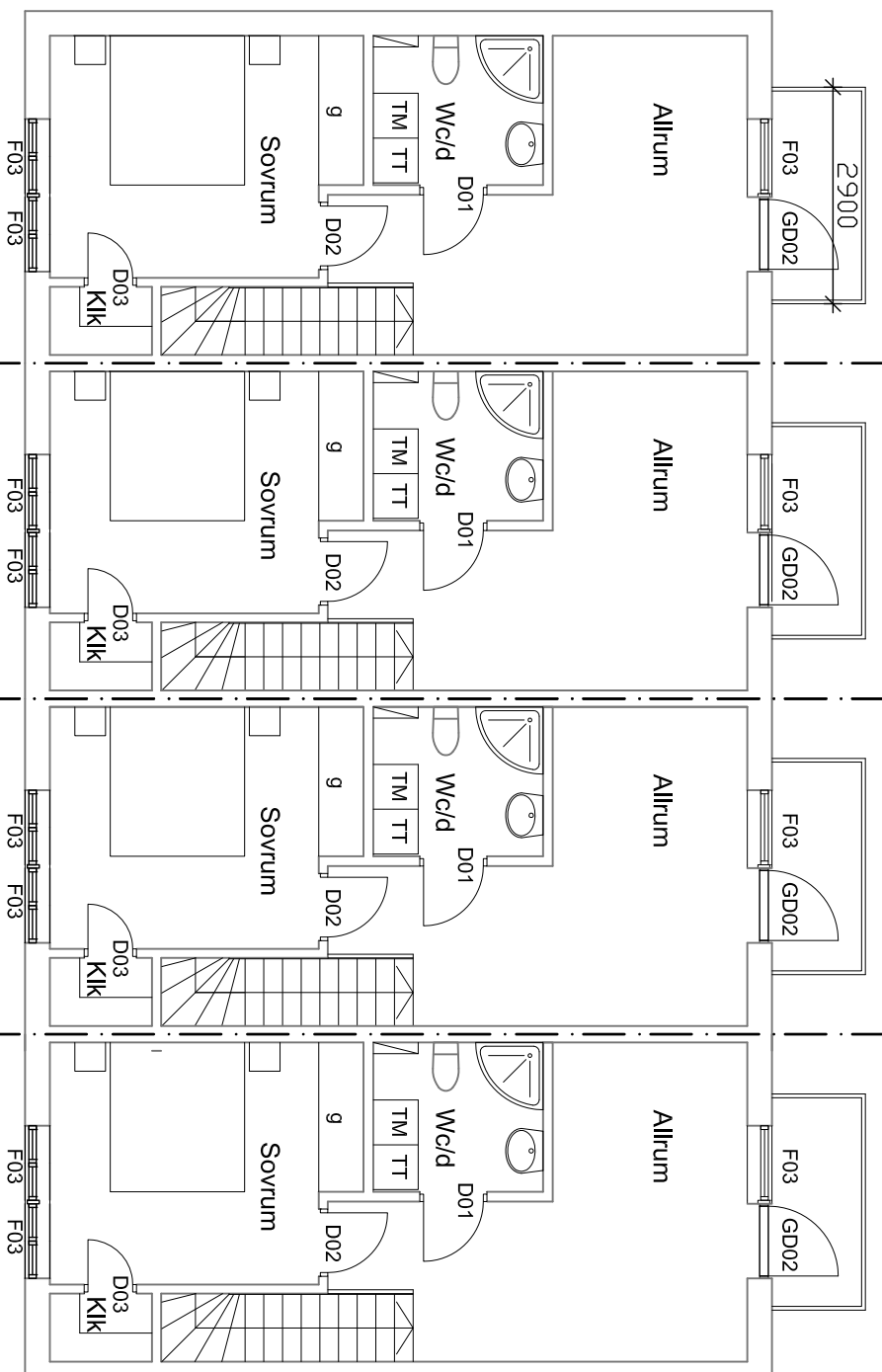
Övre plan
